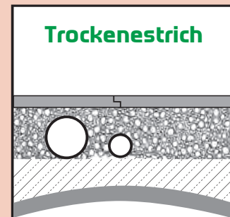
Gewölbe
